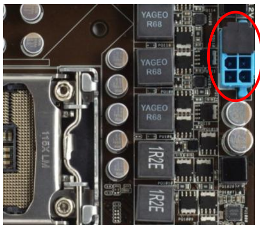
4+4 Pin Socket
